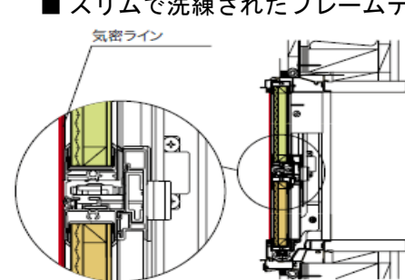
気密性能を安定させる フラットな気密ライン
